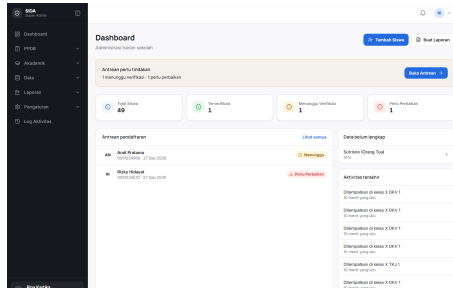
Desktop 1440×900
