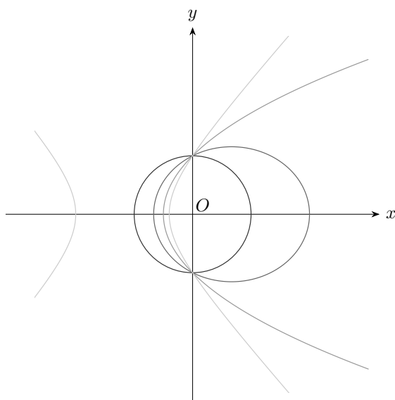
图 B-3: 固定 p = 1 时, 不同离心率对应的轨迹
