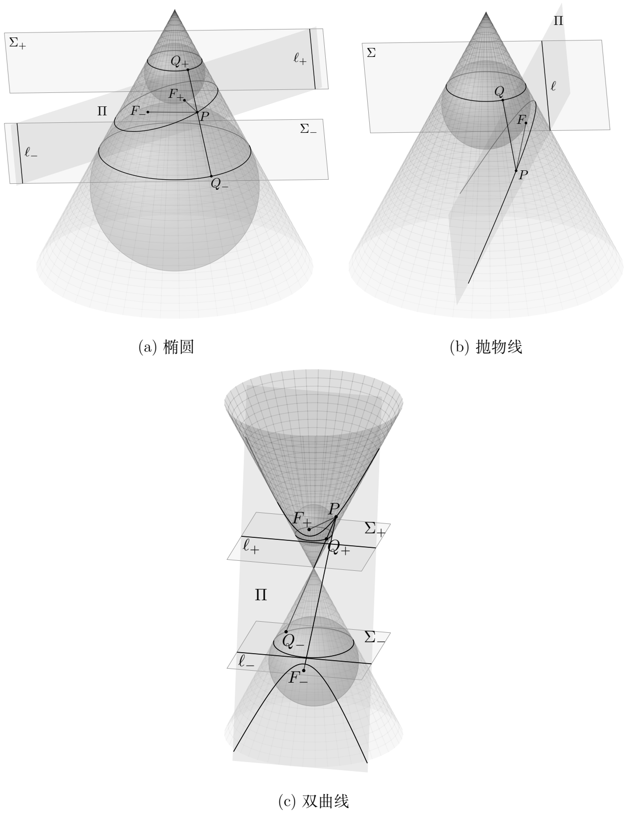
图 B-9: 椭圆、抛物线与双曲线截面中的 Dandelin 球
