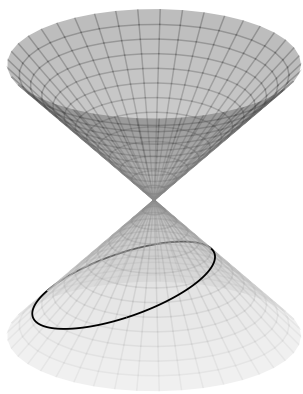
(a) 椭圆截线
