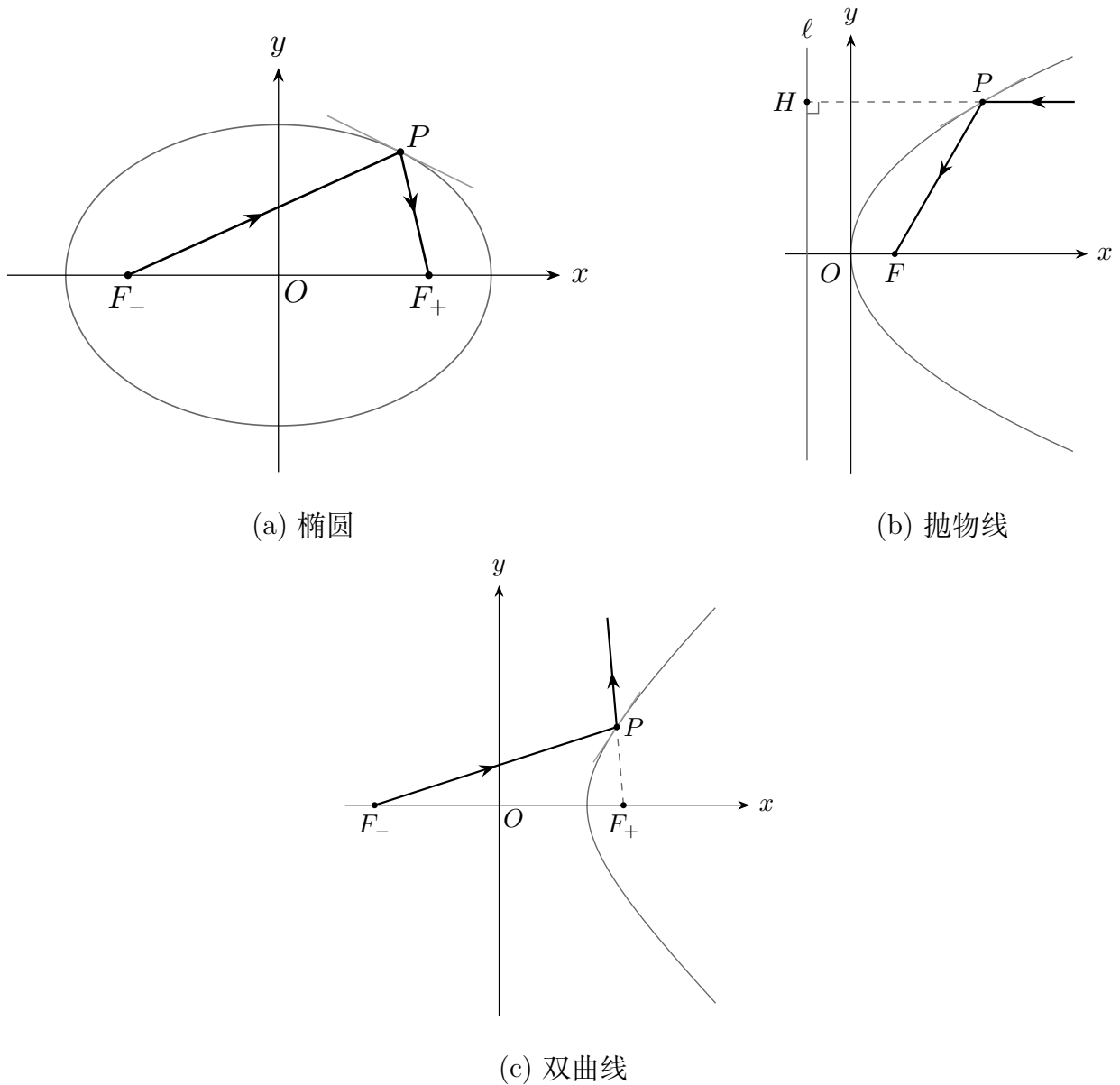
图 B-13: 椭圆、抛物线与双曲线的反射性质
