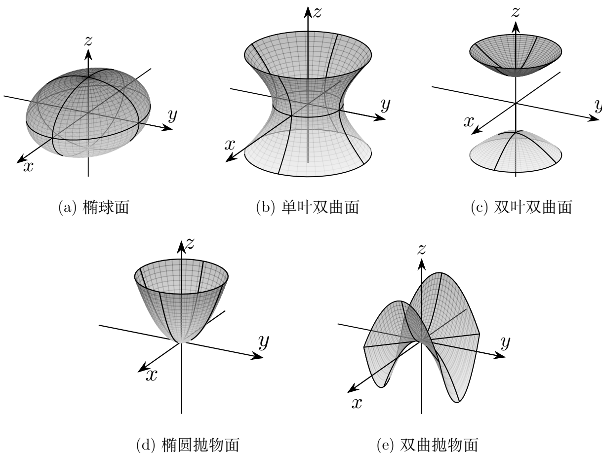
图 B-12: 五种非退化实二次曲面的典型形状
