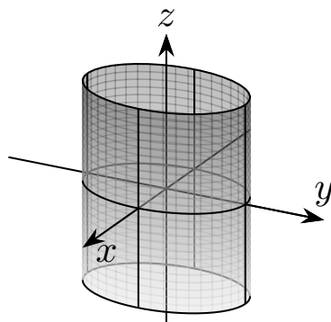
(b) 椭圆柱面
