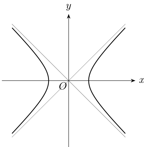
图 B-7: 标准双曲线及其两条渐近线
