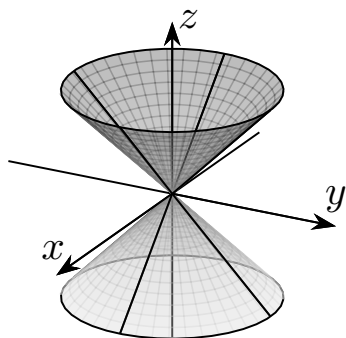
图 B-8: 双圆锥的整体形状
