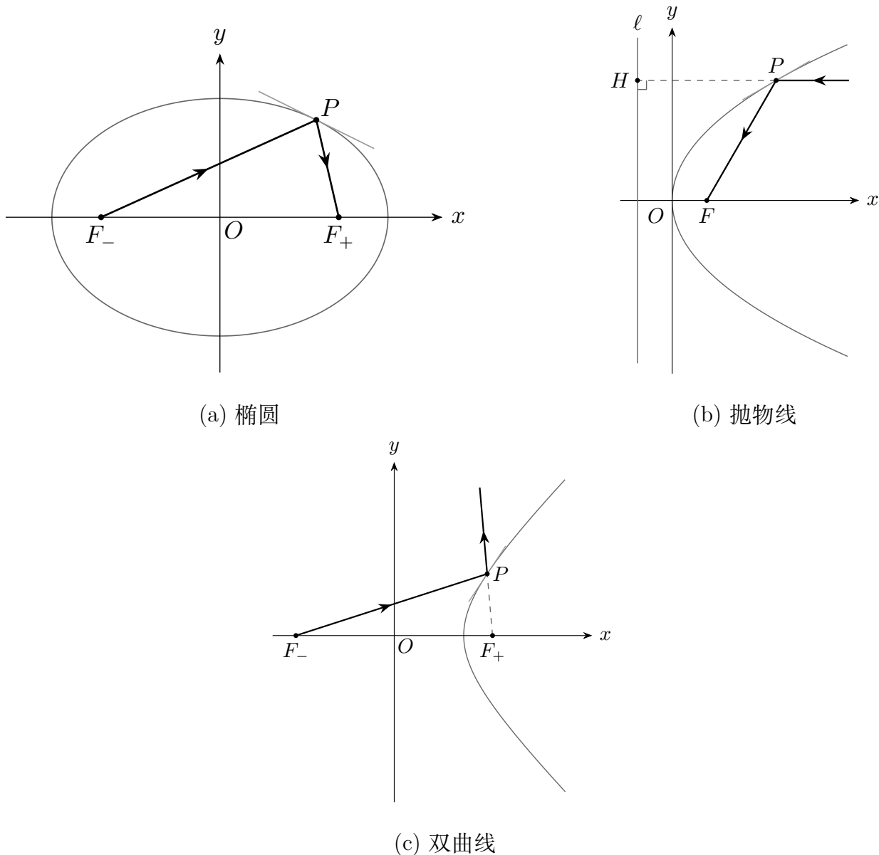
图 B-14: 椭圆、抛物线与双曲线的反射性质
