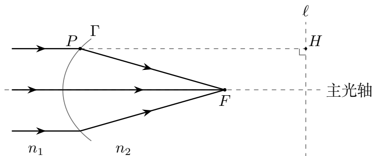
(a) 物点到像点的精确折射
