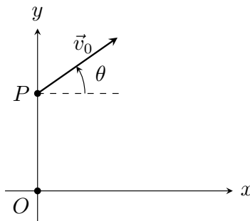
图 A-1: 炮弹从高度 h 处发射时的初速度方向示意图
