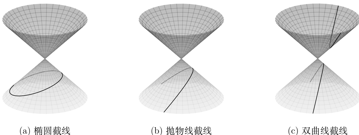
图 B-9: 截平面相对于圆锥母线的倾斜程度不同时，双圆锥的截线
