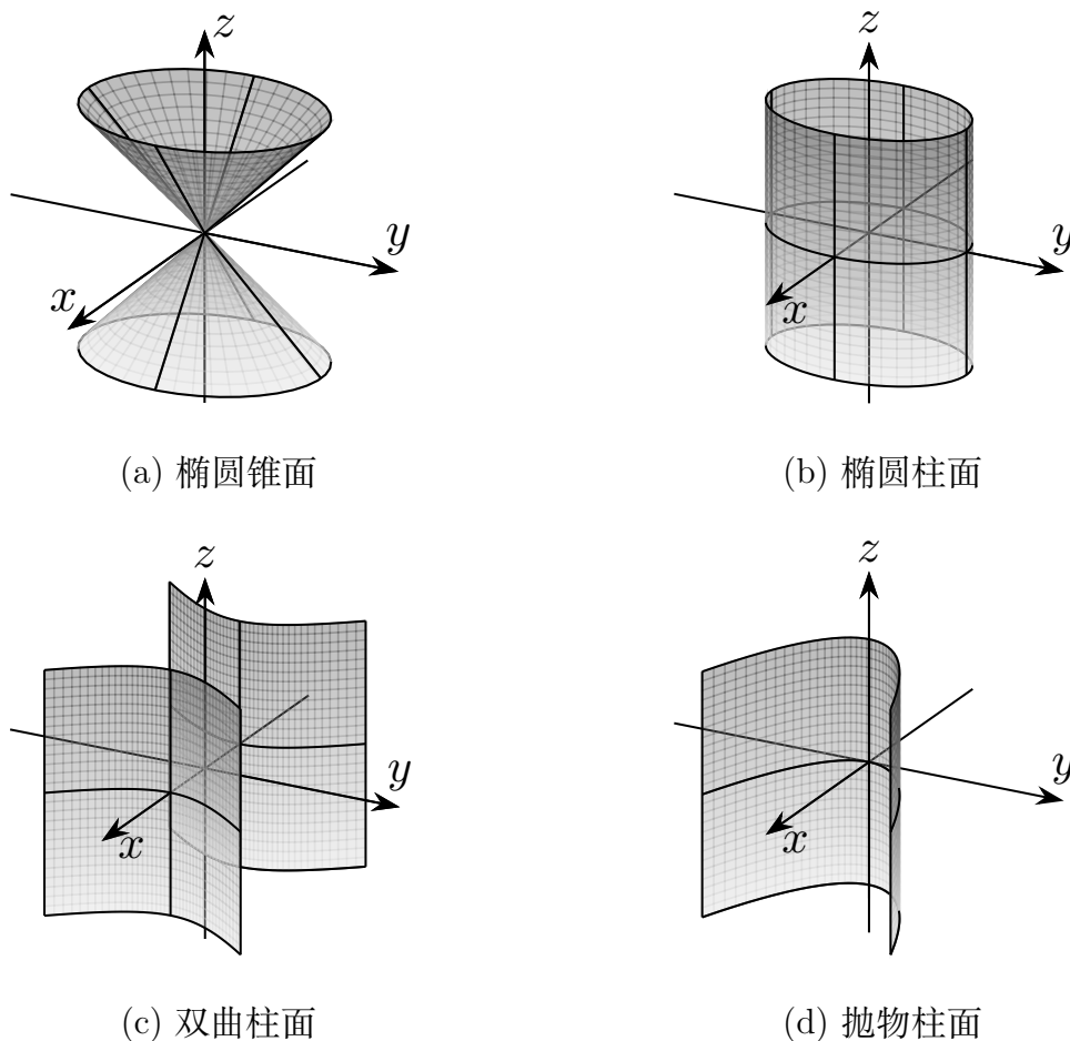
图 B-13: 四种常见的退化实二次曲面
