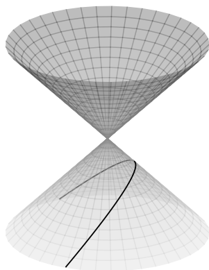
(b) 抛物线截线
