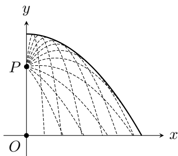
图 A-3: 不同发射方向对应的抛物线族及其上方边界
