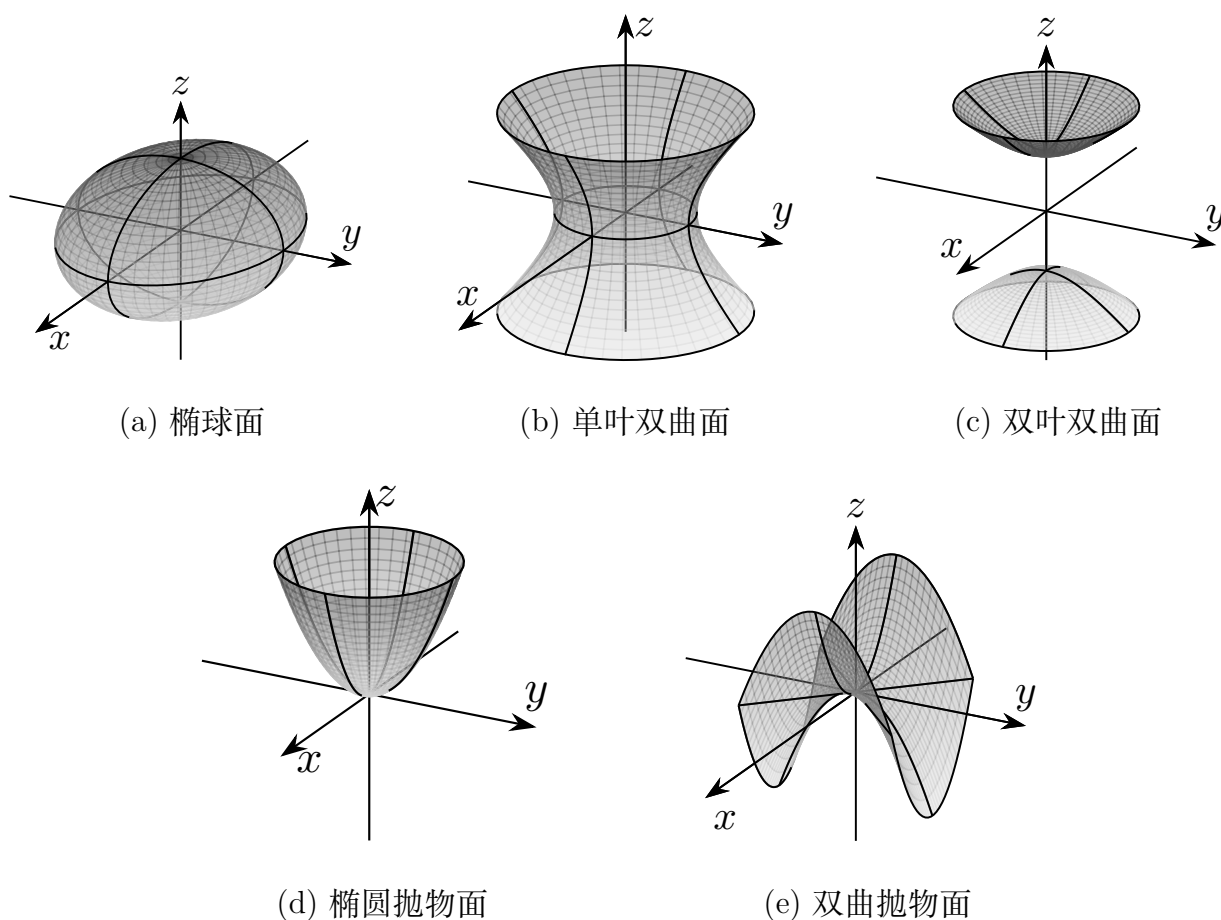
图 B-4: 五种非退化实二次曲面的典型形状
