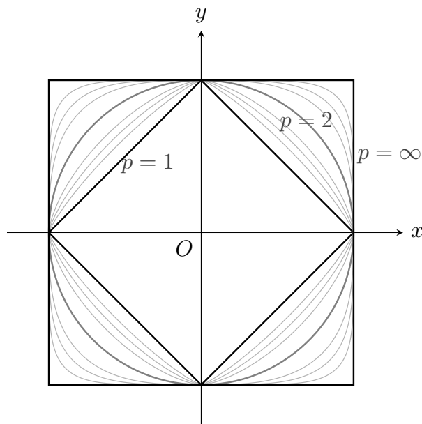
图 C-8: \mathbb{R}^2 中若干 p -范数的单位圆；其中只有 p = 2 的单位圆在任意旋转下保持不变
