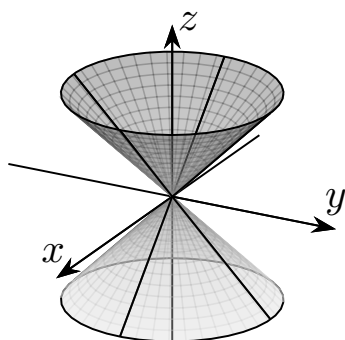
图 B-4: 双圆锥的水平截面与经过轴线的截面
