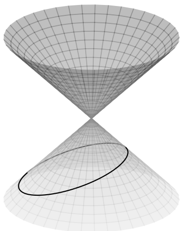
(a) 椭圆截线
