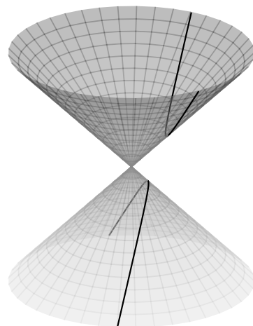
(c) 双曲线截线
