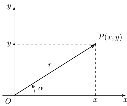
图 B-2: 点 P 的坐标表示 (图中画出的是 0 < \alpha < \frac{\pi}{2} 的情形)
