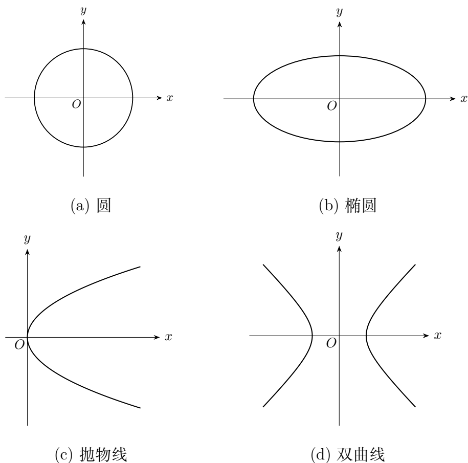
图 B-1: 四种常见的非退化二次曲线
