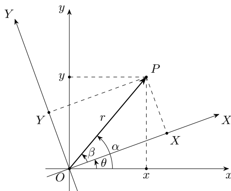
图 B-3: 点 P 在旋转前后两个坐标系中的表示 (图中角度仅用于示意)
