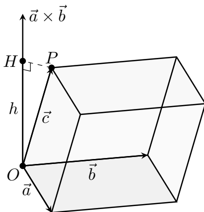
图 D-3: 平行六面体的底面积、正法向与有向高
