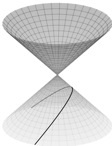
(b) 抛物线截线
