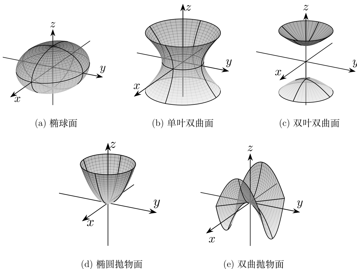
图 B-10: 五种非退化实二次曲面的典型形状
