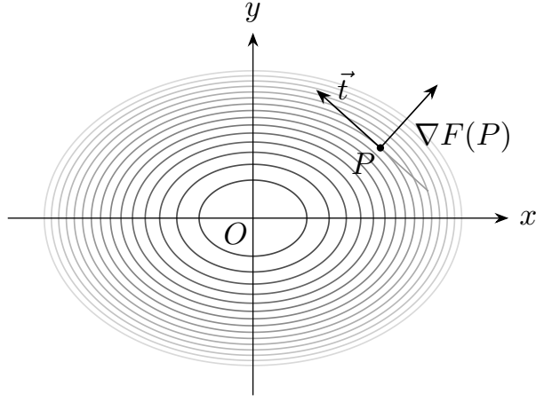
图 C-9: 水平集的切方向与梯度方向
