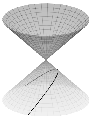
(b) 抛物线截线
