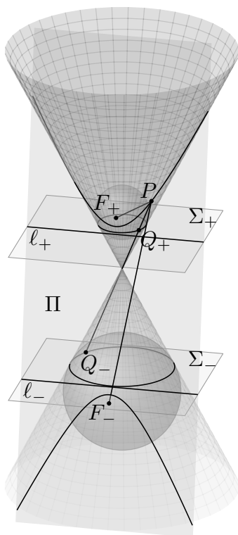
(c) 双曲线
