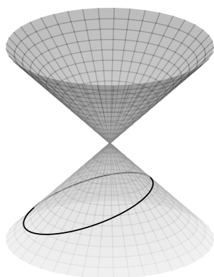
(a) 椭圆截线
