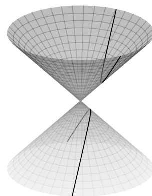
(c) 双曲线截线
