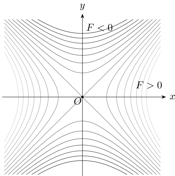
图 C-8: 鞍点附近的双曲线水平集
