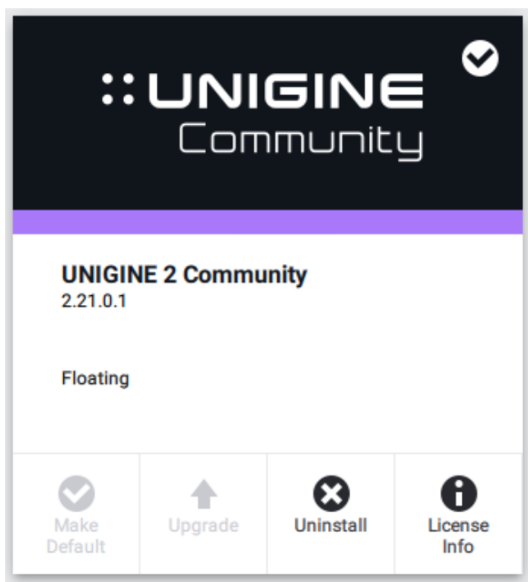
Рис. 3: Используемое SDK
