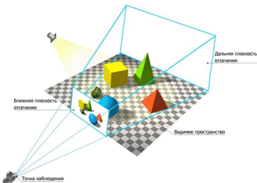
Рис. 2: Перспективная проекция
