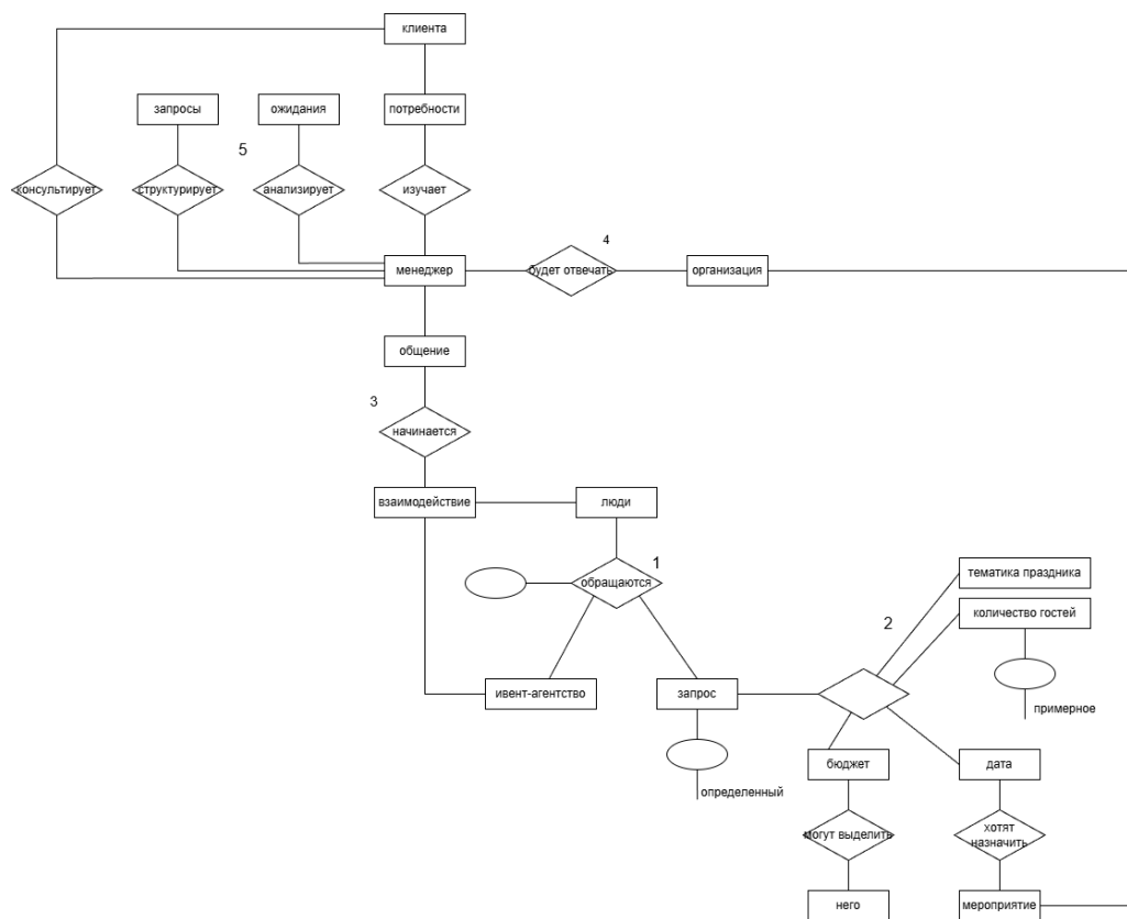
Рис. 1. ER-диаграмма
