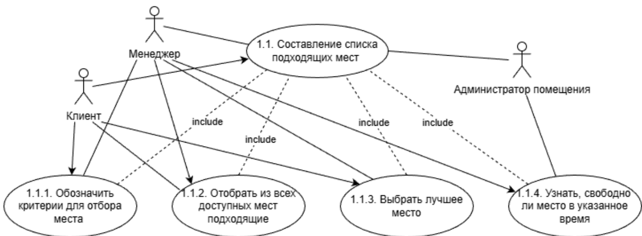
Рис. 3. Use-case диаграмма
