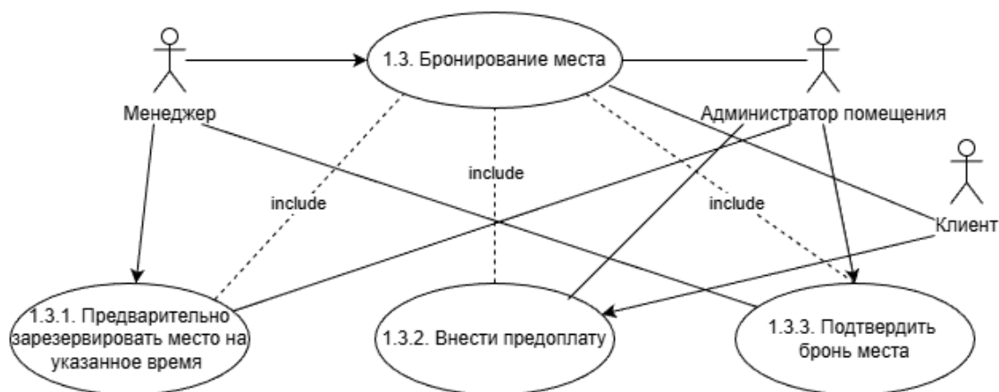
Рис. 5. Use-case диаграмма
