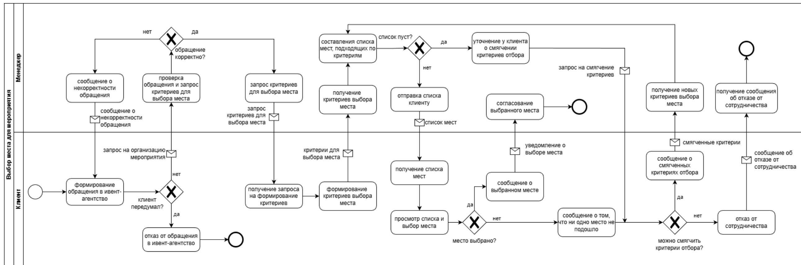
Рис. 6. BPMN-диаграмма
