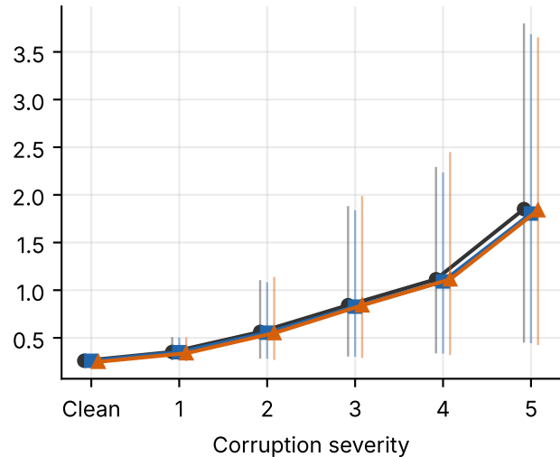
NLL (nats)
