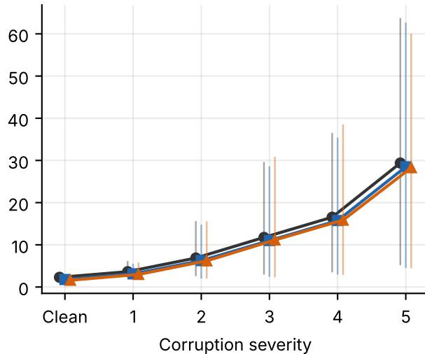
ECE (%)
