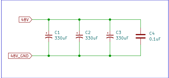
Decoupling Caps
