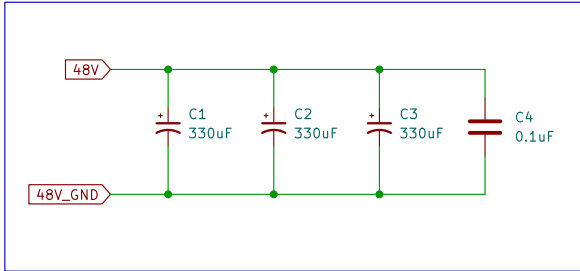
Decoupling Caps
