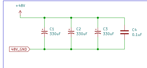
Decoupling Caps
