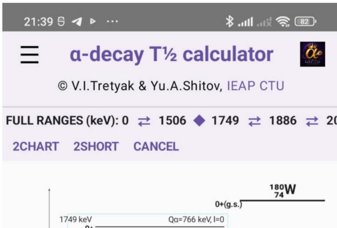
Рисунок 9. Режим FULL RANGES: вибраний енергетичний діапазон схеми альфа-розпаду ^{180}\text{W} \rightarrow ^{176}\text{Hf} .
