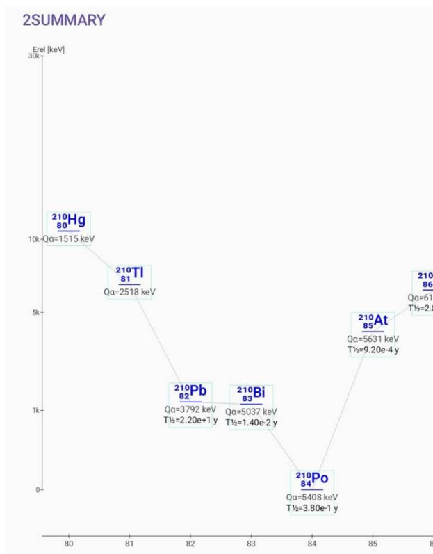
Рисунок 8. Приклад діаграми шару А = 210.
