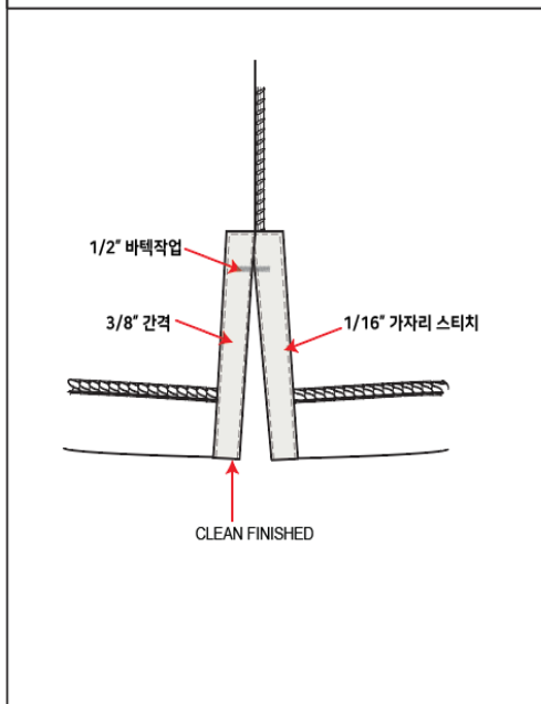
사이드벤트 사양 (내부 사양)
