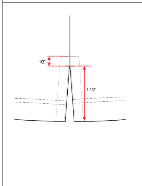
사이드벤트 사양 (외부 사양)
