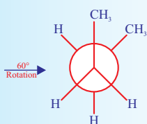
Gauche (more stable)
