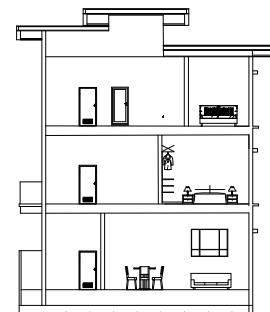
SECTION THRU -- X SCALE: 1:150
