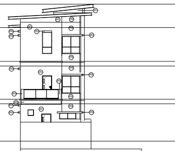
8 A 2 LEFT SIDE ELEVATION SCALE: 1:150
