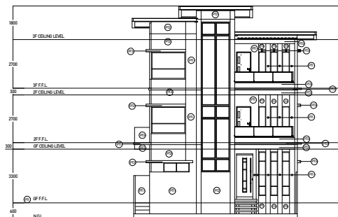
7 A 2 FRONT ELEVATION SCALE: 1:150
