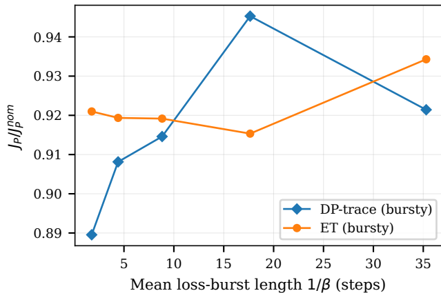
(d) Bursty losses
