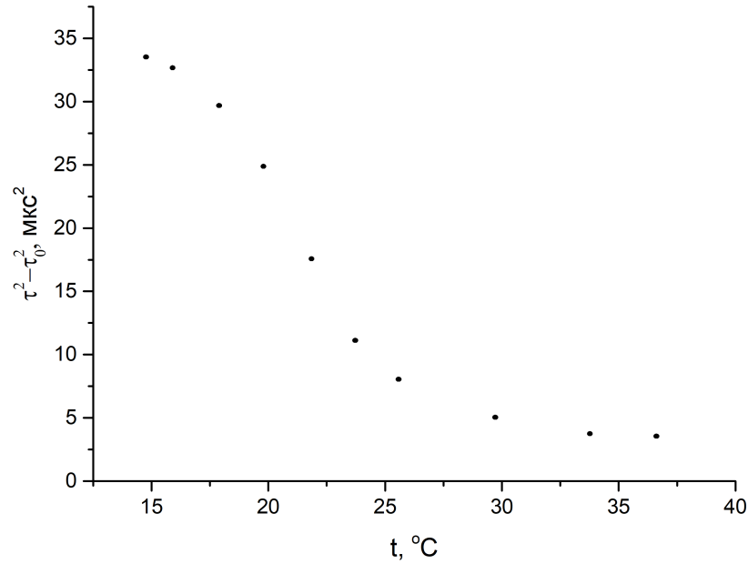
Рис. 3: Зависимость \tau^2 - \tau_0^2 = f(t)
