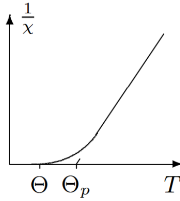
Рис. 1: Зависимость обратной величины магнитной восприимчивости от температуры
