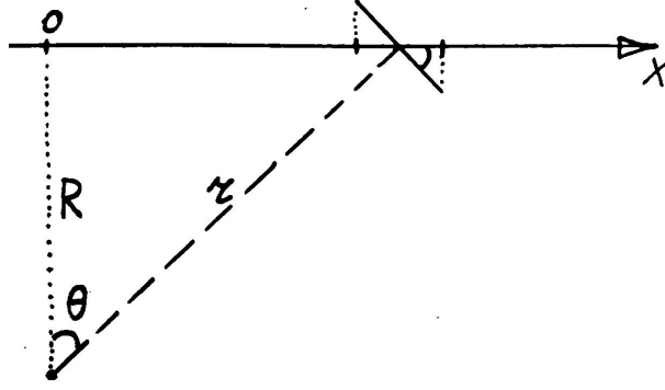
Рис. 1: Геометрия напыления
