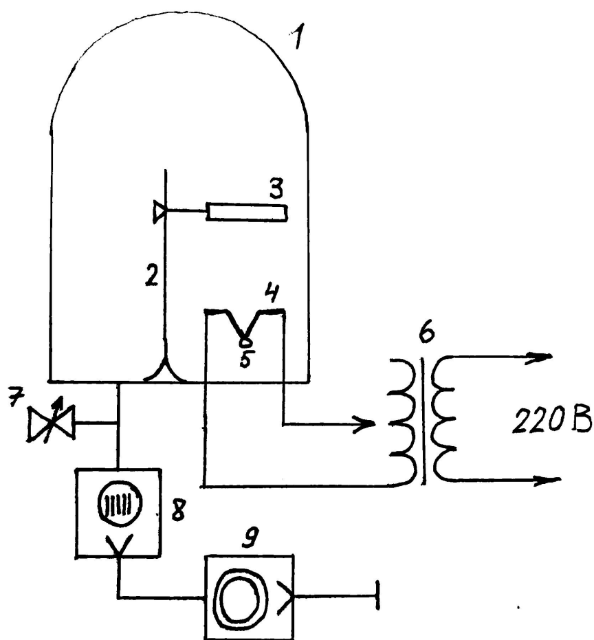
Рис. 3: Упрощённая схема установки: 1 – вакуумный колпак, 2 – штатив, 3 – стеклянная пластинка, 4 – вольфрамовый испаритель, 5 – образец алюминия, 6 – трансформатор, 7 – натекатель, 8 – турбомолекулярный насос, 9 – форвакуумный насос
