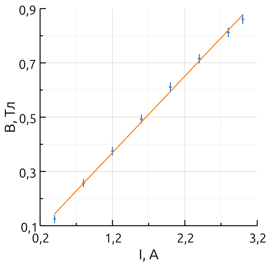
Рис. 3: Градуировка электромагнита B(I)
