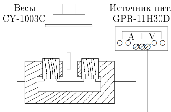
Рис. 1: Схема установки
