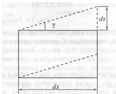
Рис. 1: Деформация сдвига
