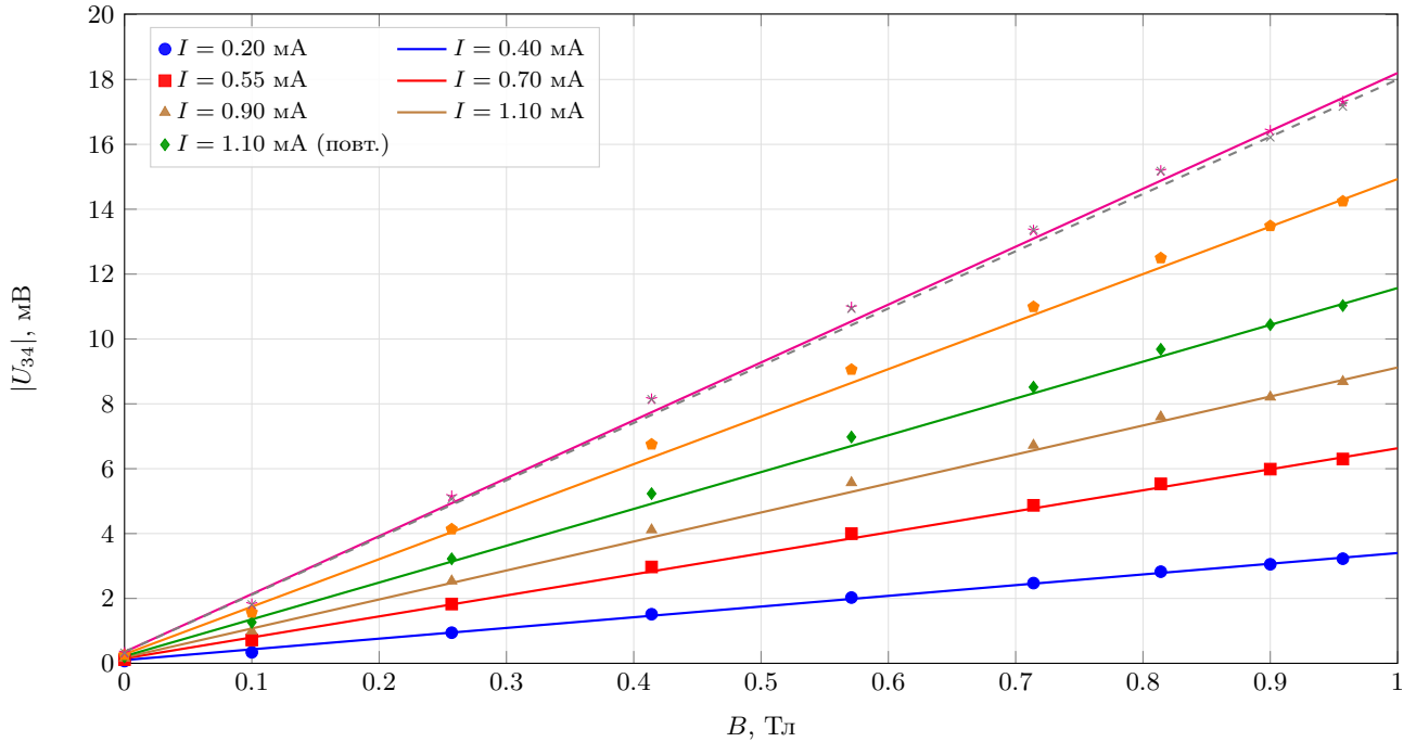
Рис. 5: Семейство зависимостей ЭДС Холла от индукции магнитного поля при различных токах через образец
