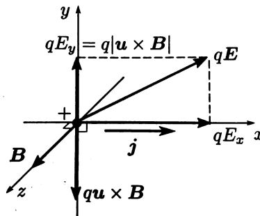
Рис. 1: Силы, действующие на положительный носитель заряда в проводнике в магнитном поле
