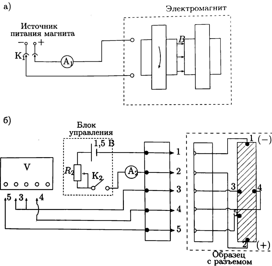
Рис. 3: Схема установки
