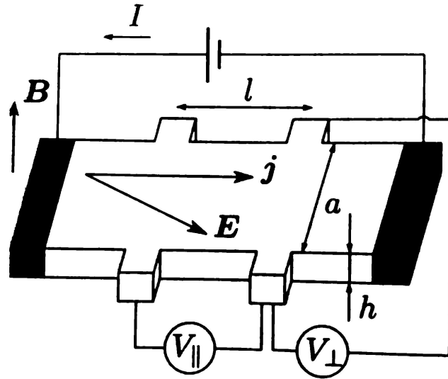
Рис. 2: Мостик Холла
