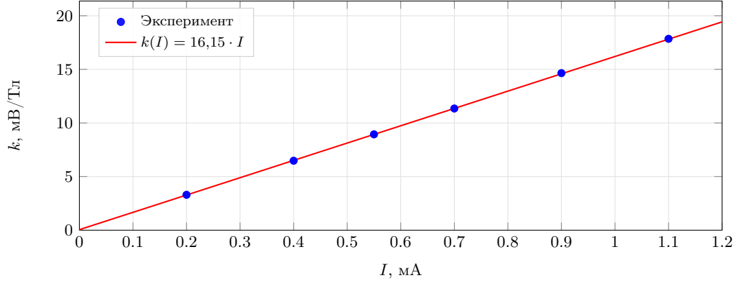
Рис. 6: Зависимость углового коэффициента от тока
