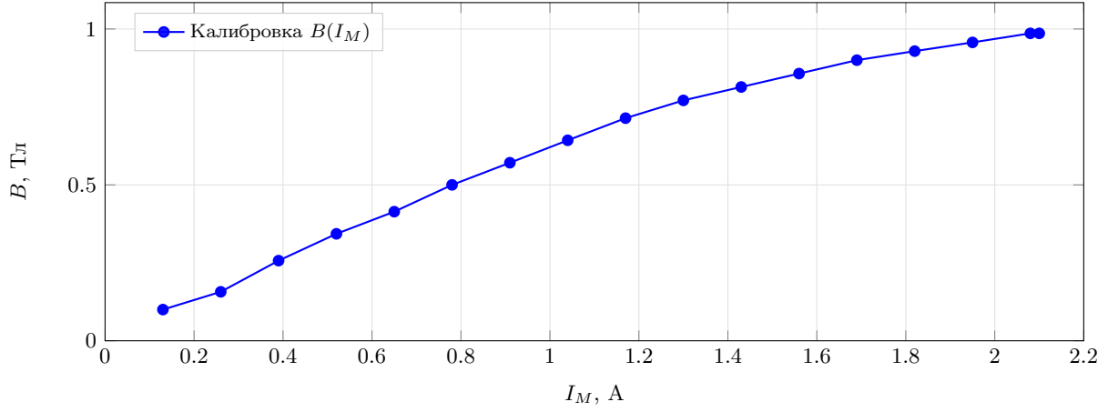
Рис. 4: График калибровки электромагнита
