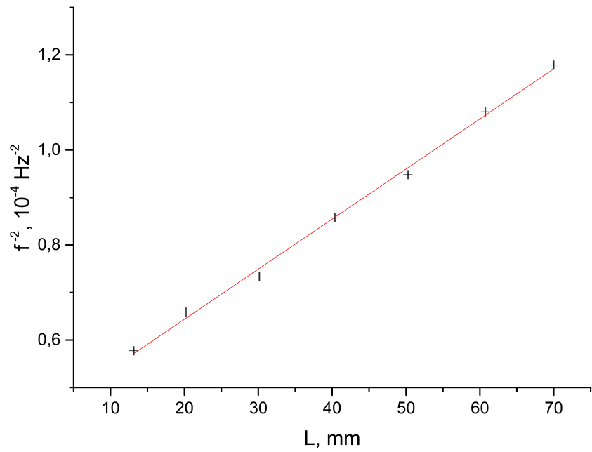
Рис. 6.2: График зависимости f^{-2}(L)
