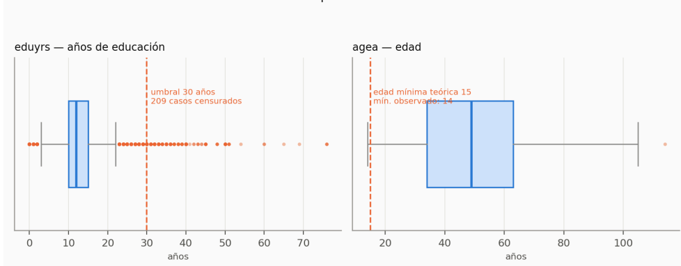
Figura 1. Distribución de eduys y agea antes de la depuración. Los puntos naranjas señalan valores atípicos; las líneas discontinuas, los umbrales de referencia.
