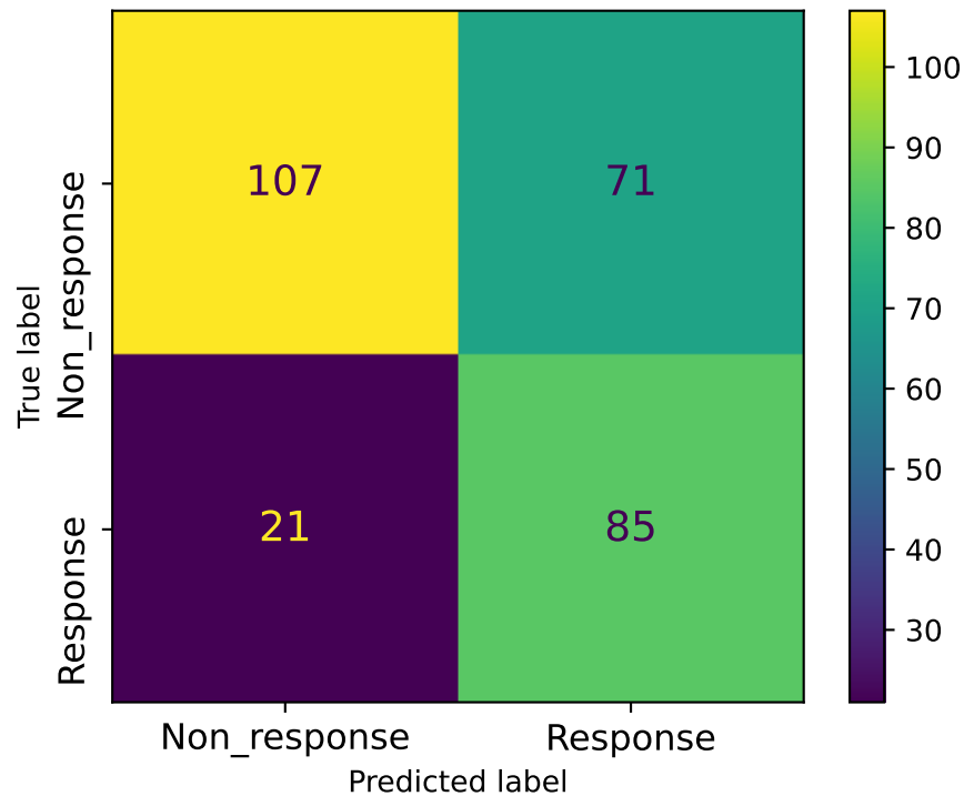
Matriz de confusión (umbral=0.19)
