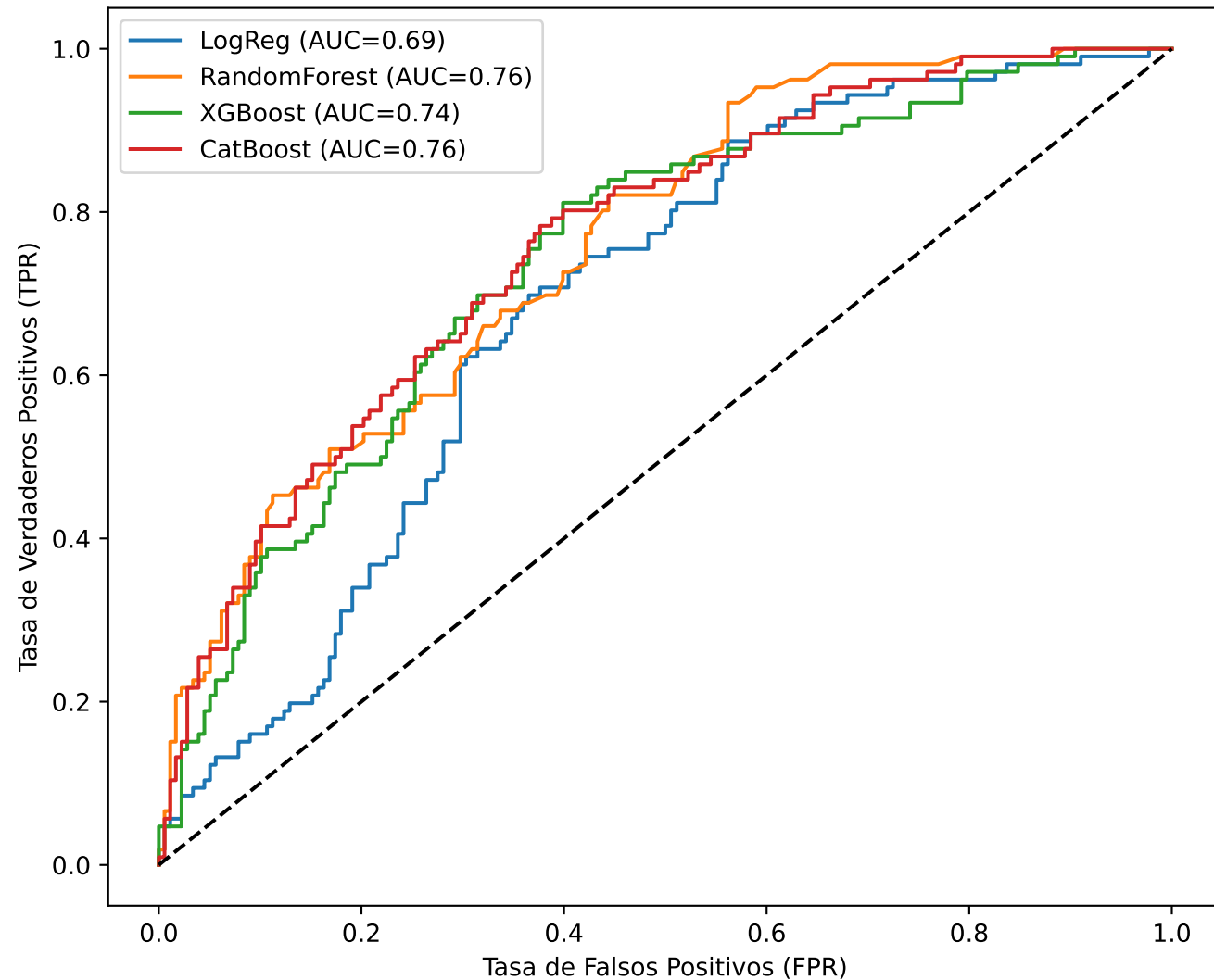
Curvas ROC - Todos los modelos
