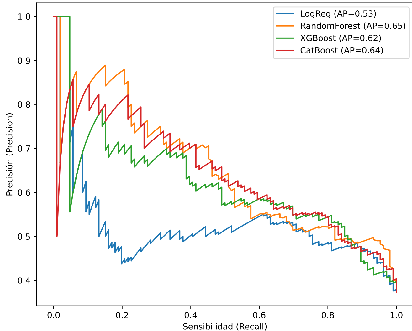
Curvas Precision-Recall - Todos los modelos
