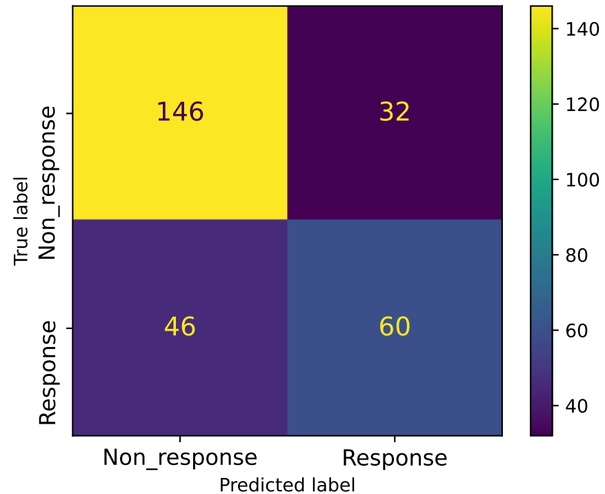
Matriz de confusión (umbral=0.5)
