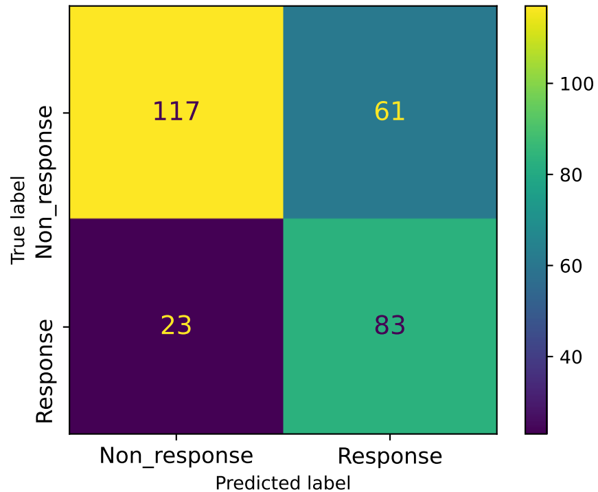
Matriz de confusión (umbral=0.41)
