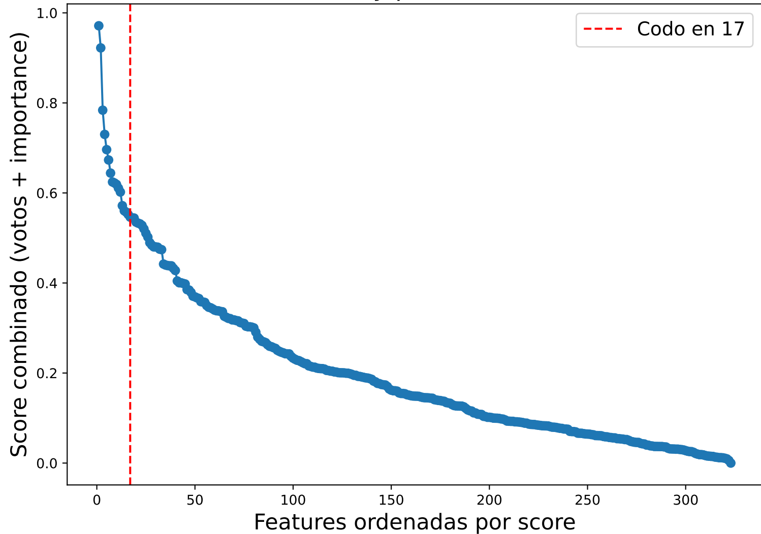
Curva de scores y punto de corte (codo)
