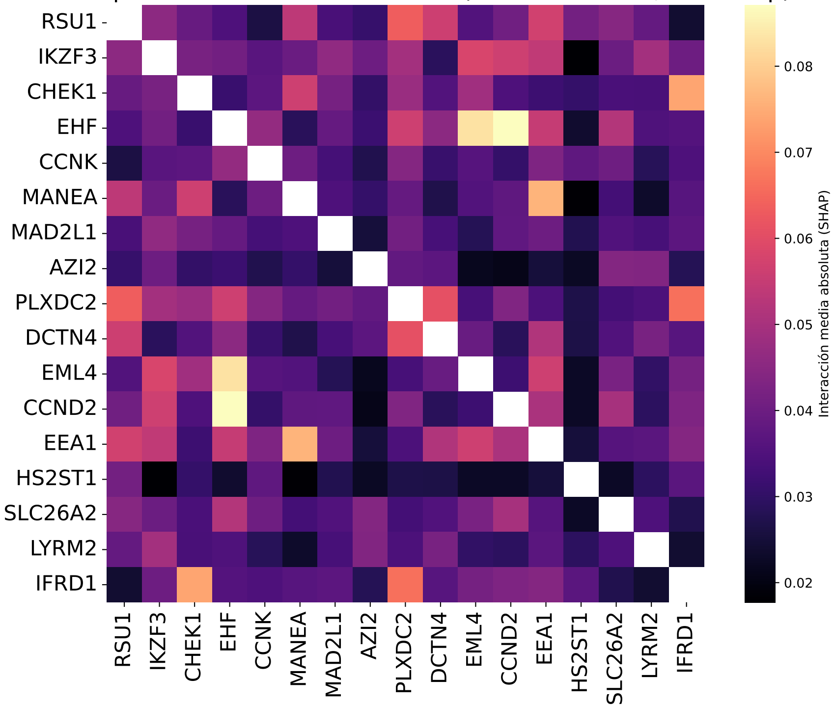
Heatmap de SHAP interaction values (media absoluta, bootstrap)
