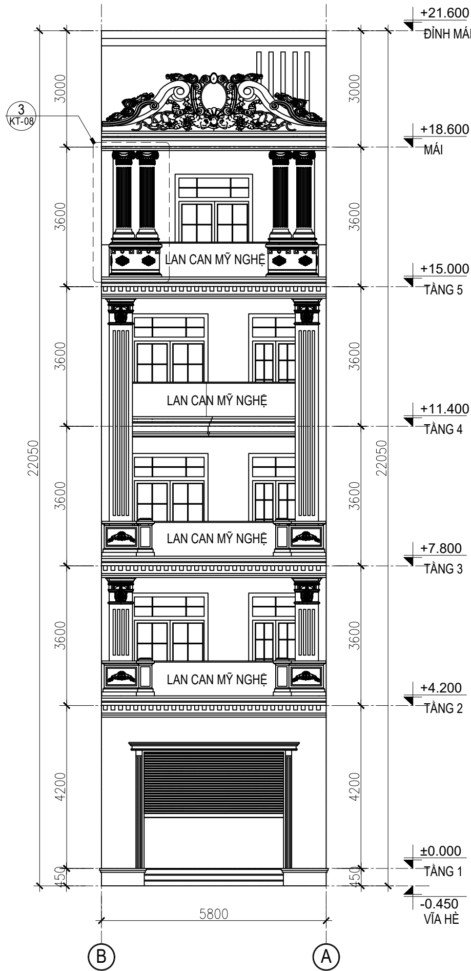
MẶT ĐỨNG TRỤC B-A
