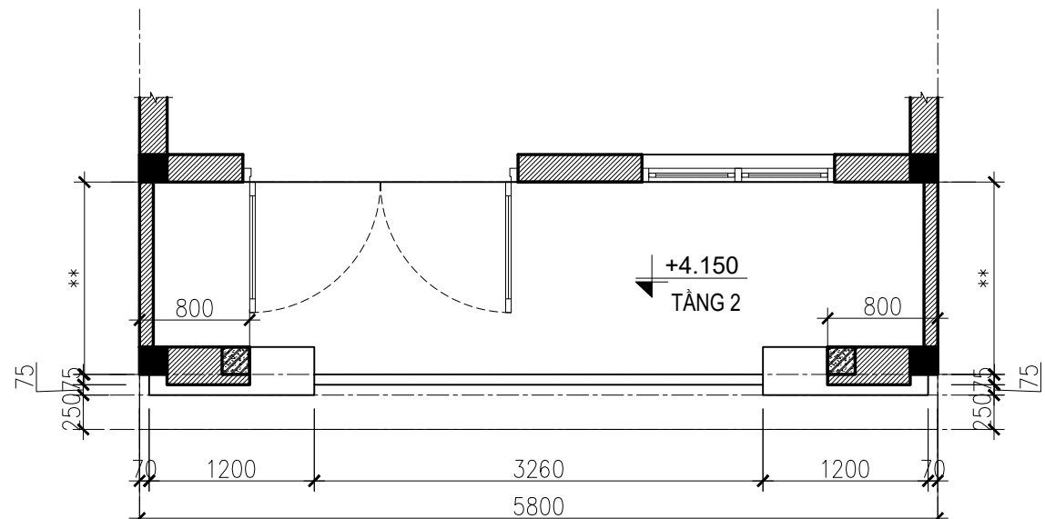
BAN CON TẦNG 2
