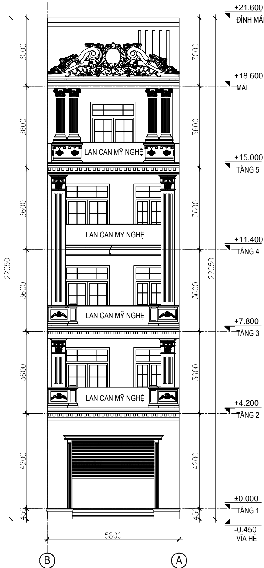
MẶT ĐỨNG TRỰC B-A
