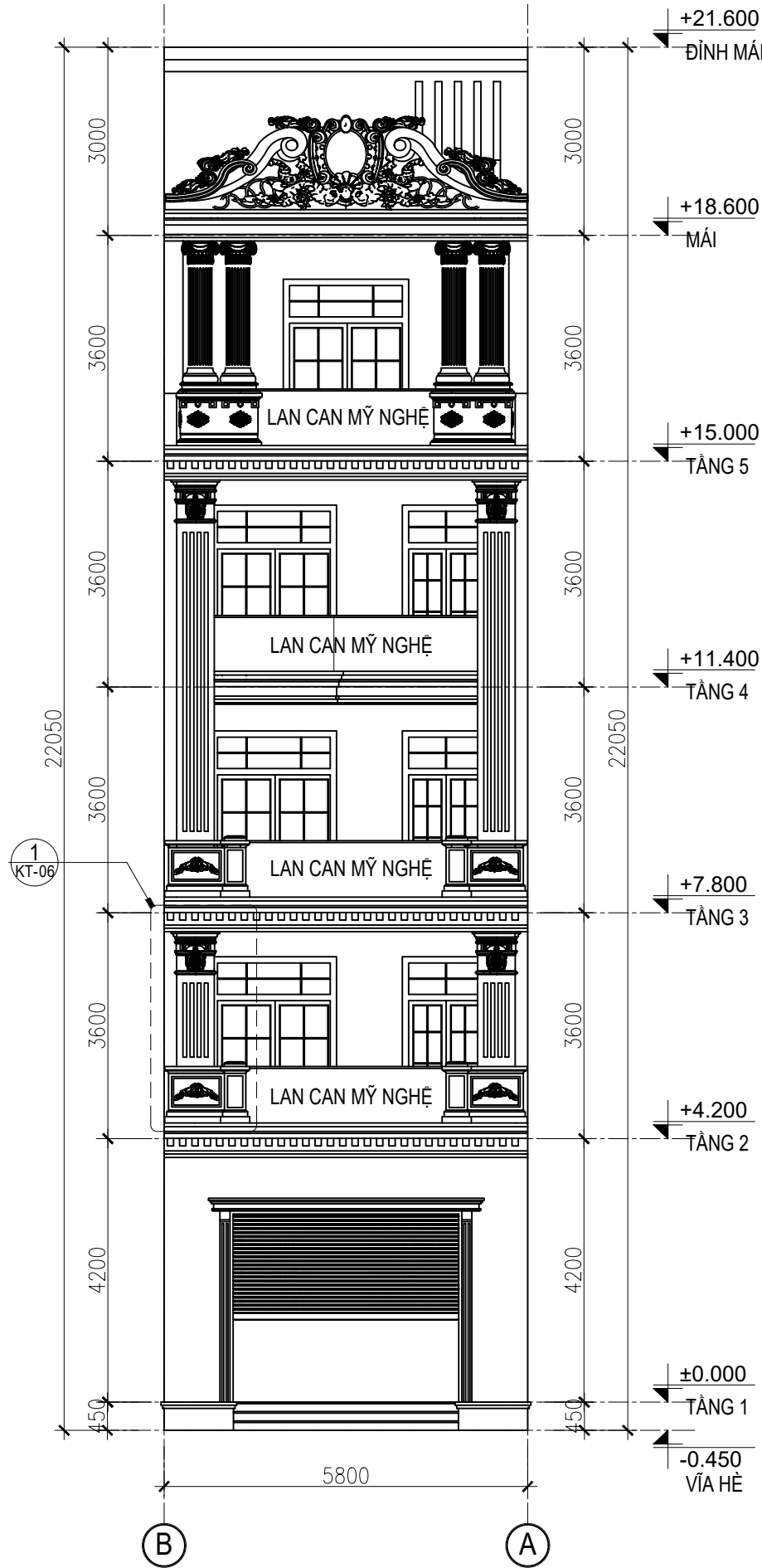
MẶT ĐỨNG TRỰC B-A
