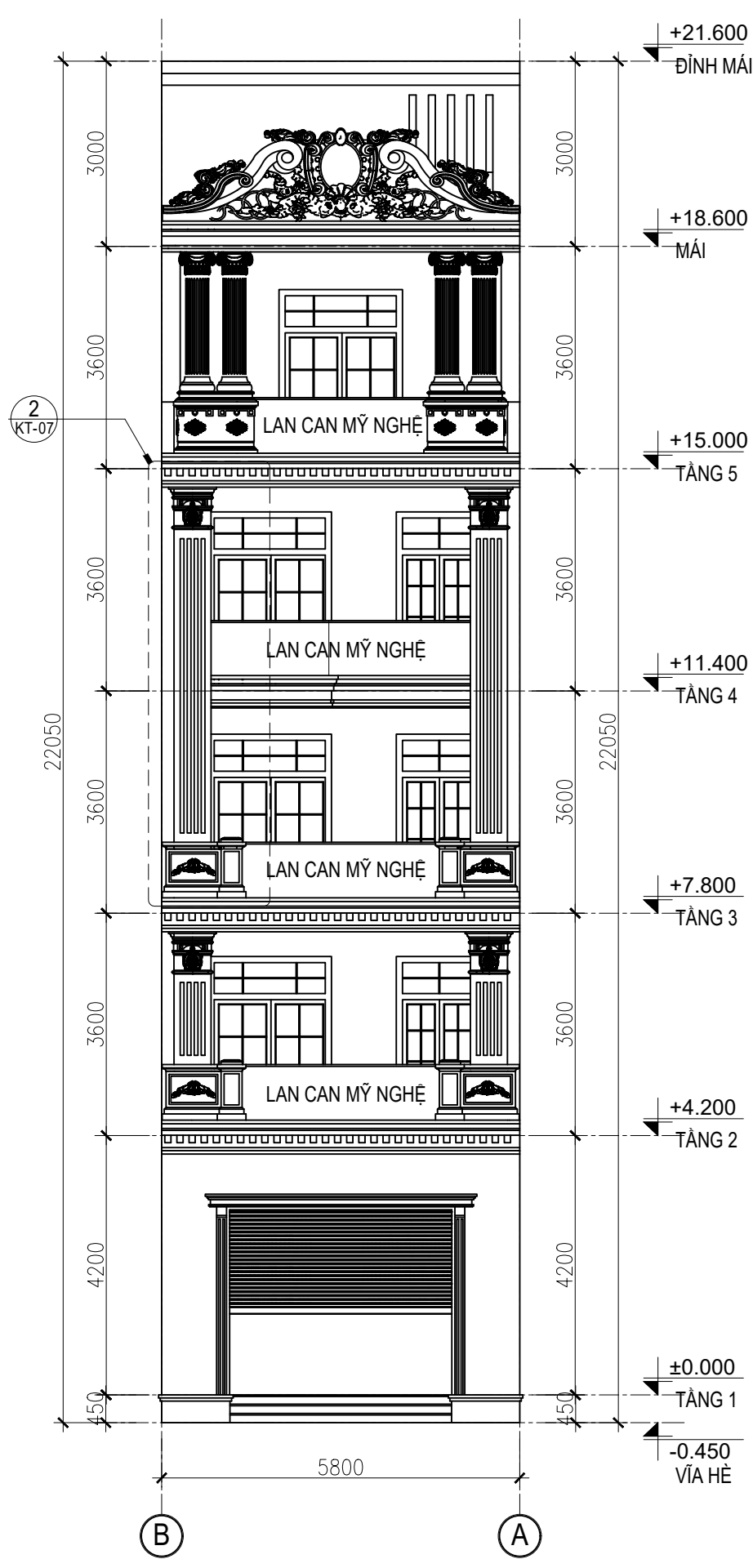
MẶT ĐỨNG TRỤC B-A TL: 1/100
