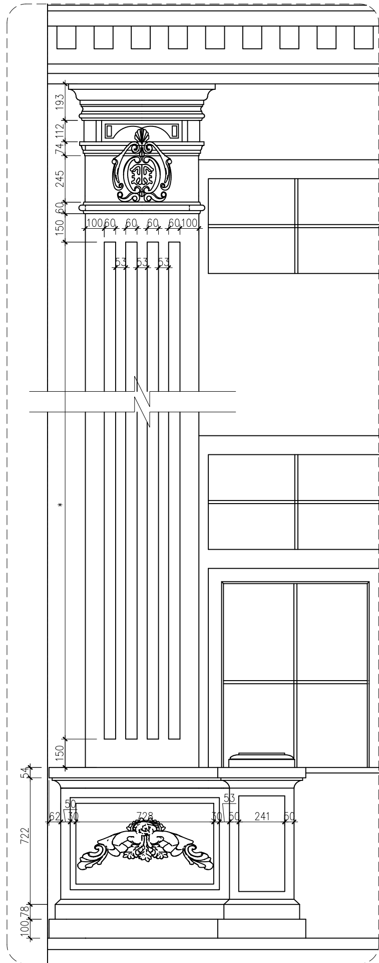
CHI TIẾT 2 TL: 1/20
