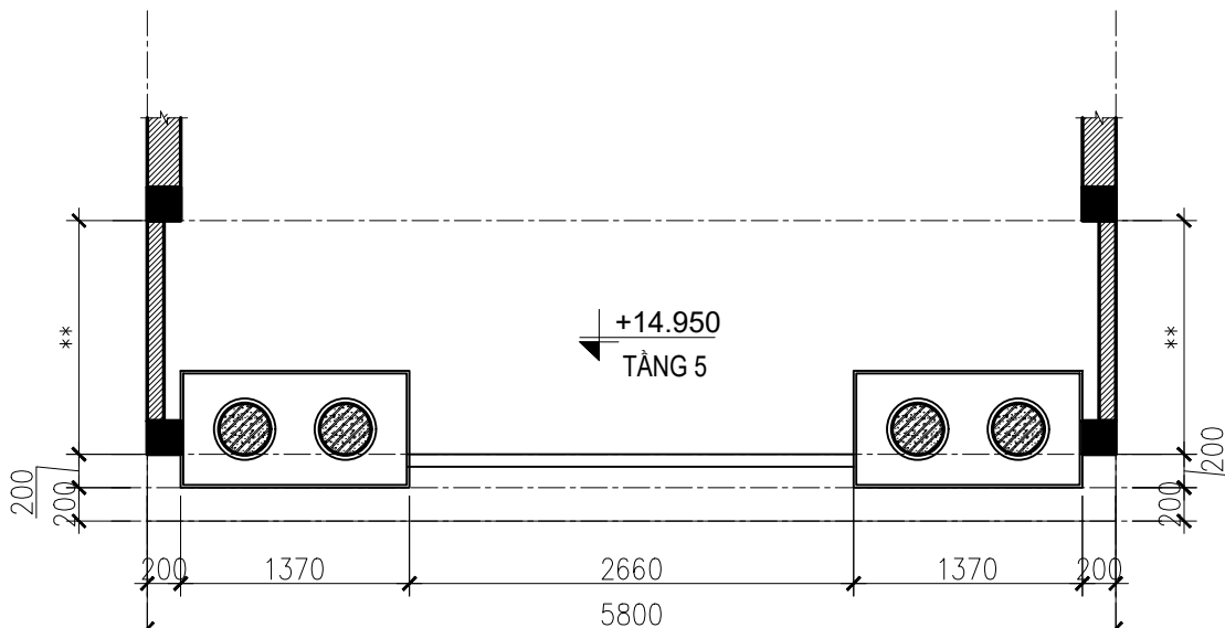
BAN CON TẦNG 5
