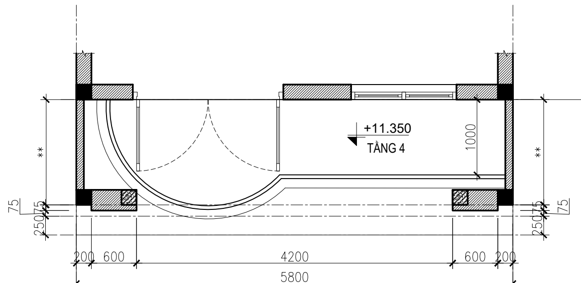
BAN CON TẦNG 4
