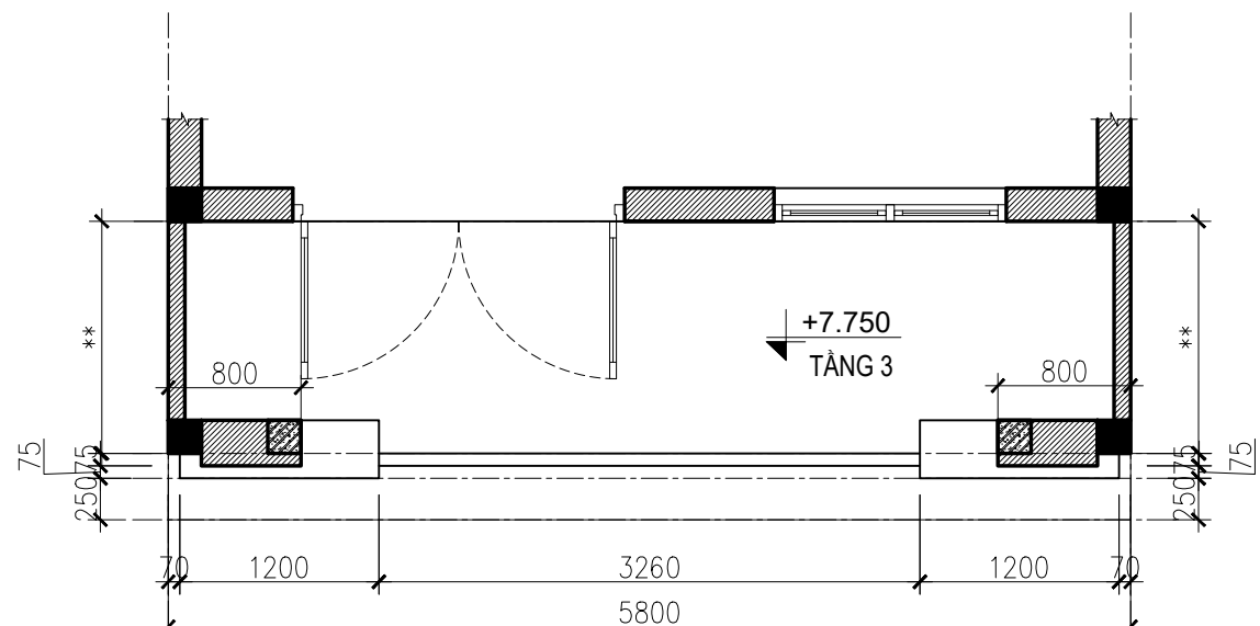
BAN CON TẦNG 3
