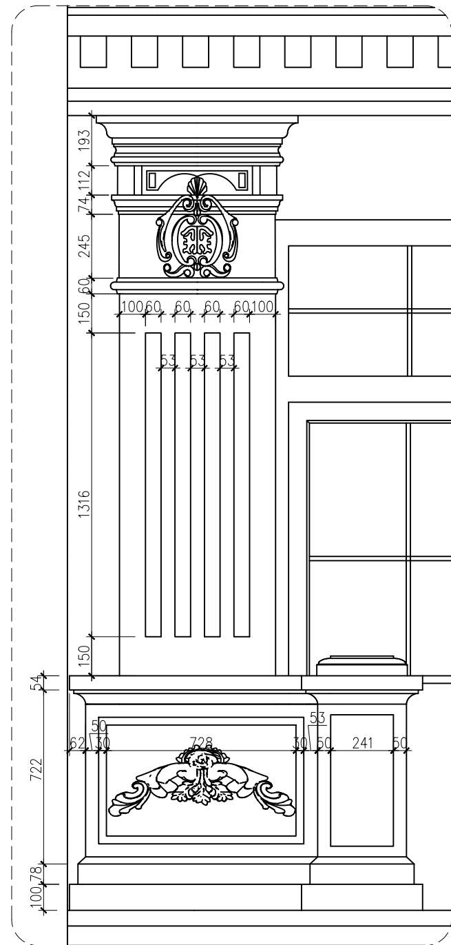
CHI TIẾT 1
