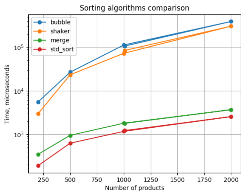
Figure 1: График времени сортировок
