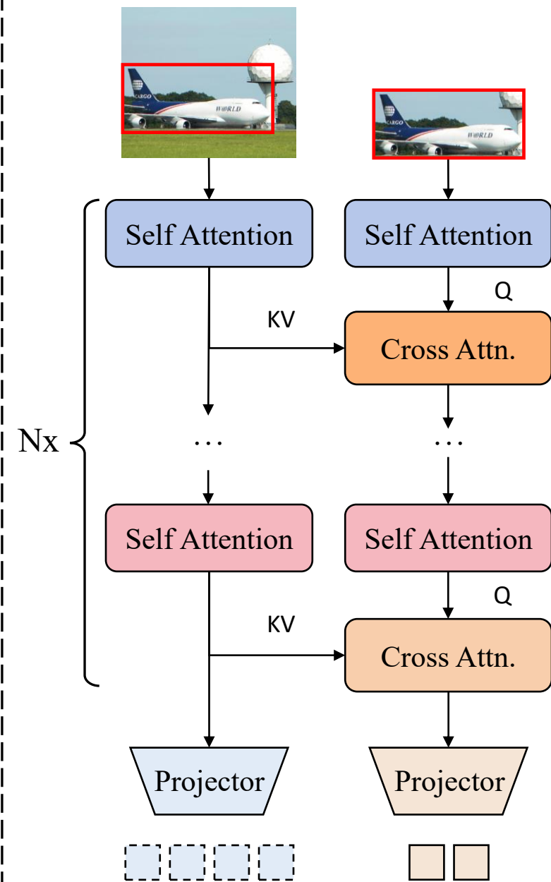
(d) LEMUR (Ours)
