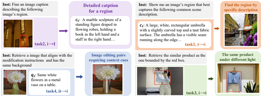
(b) FGMB Benchmark (Ours)
