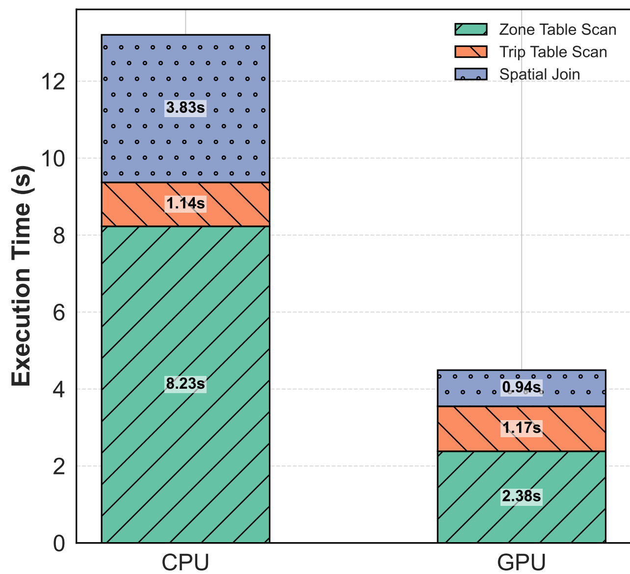
(b) Q11: CPU vs GPU Execution
