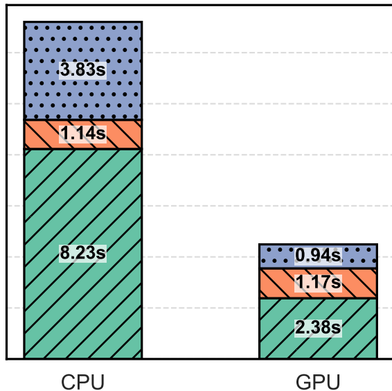
(b) Q11: CPU vs GPU
