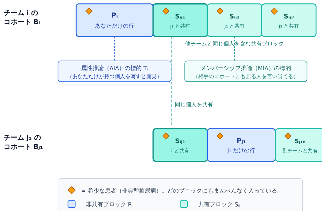
図1 図2：コホート B_i の構造。あなたがただけの行（非共有ブロック P_i = 属性推論 (AIA) の標的）と、他チームと同じ個人を含む共有ブロック S_{ij} (メンバーシップ推論の標的) からなる。
