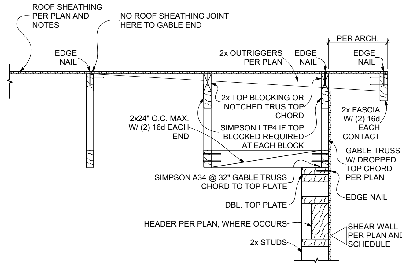
3 GABLE END DETAIL SCALE: 1" = 1'-0"
