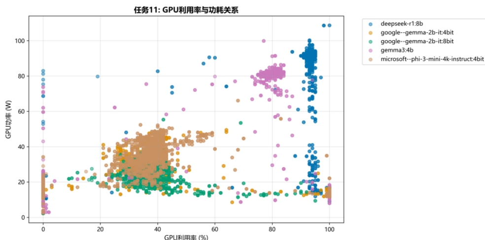
图 3-5 GPU 利用率与功耗的关联
