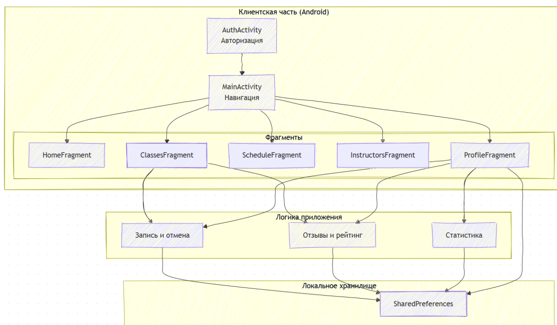
Рисунок 3.1 – Архитектурная схема приложения «Йога-студия»
