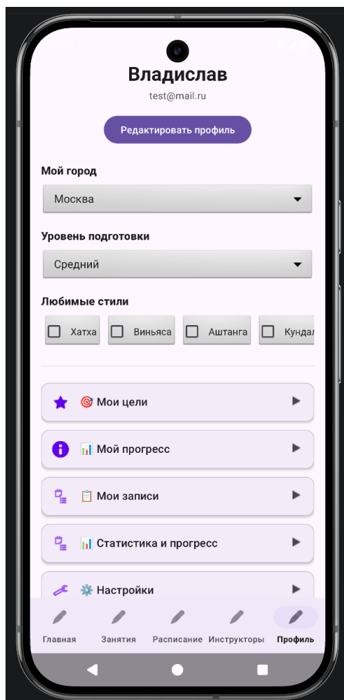
Рисунок 4.5 – Профиль пользователя
