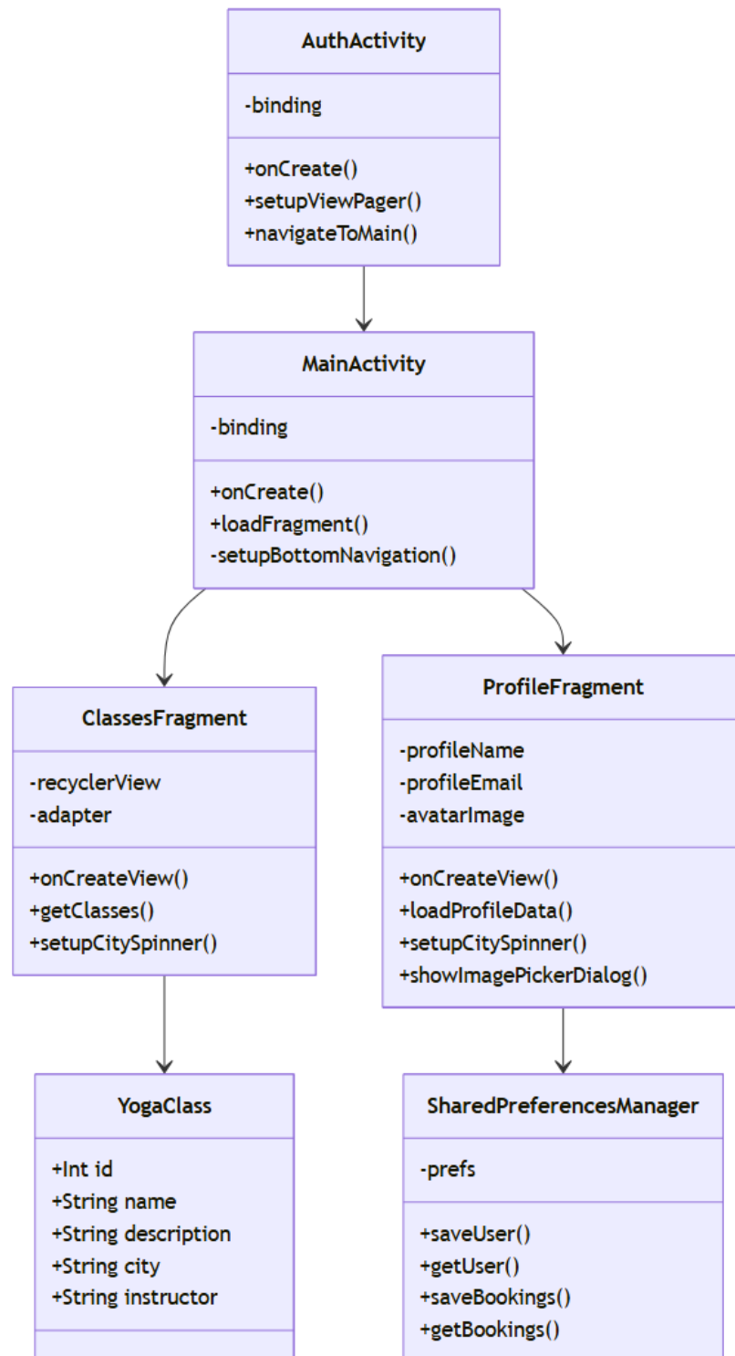
Рисунок 3.3 – Диаграмма классов
