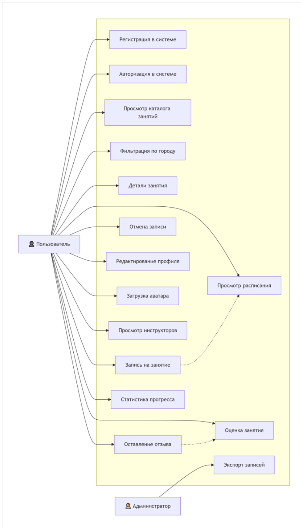
Рисунок 2.1 – Диаграмма прецедентов
