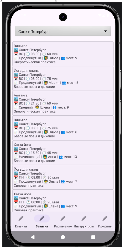
Рисунок 4.2 – Каталог занятий
