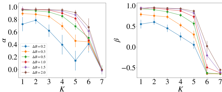
Obrázek 2: Indikátory kvantového chaosu \alpha (2) a \beta (1) v závislosti na stupni propojení K pro různé rozptyly vnějšího magnetického pole \Delta B (jsou vykresleny střední hodnoty ze 20 vzorků) s počtem uzlů N = 14 . Pro K = 7 je mříž plně propojená.
