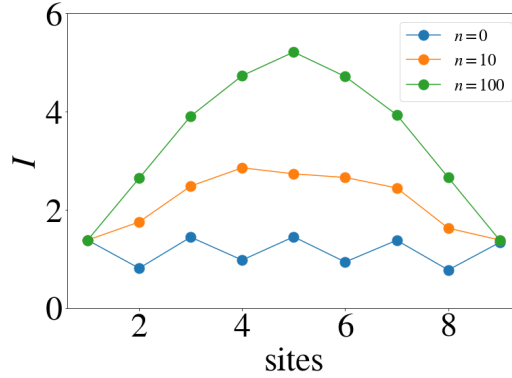
Obrázek 7: Závislost vzájemné informace souvislého úseku uzlů s jejich doplňkem na počtu uzlů v úseku řetízku pro N = 10 , \Delta B = 0,2 .
