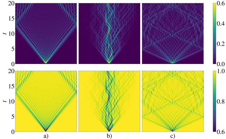
Obrázek 4: Konturové grafy entropie (nahore) a lokální magnetizace (dole) s parametry N = 100 pro a) K = 1 , \Delta B = 0 , b) K = 1 , \Delta B = 1 a c) K = 2 , \Delta B = 0,0 .
