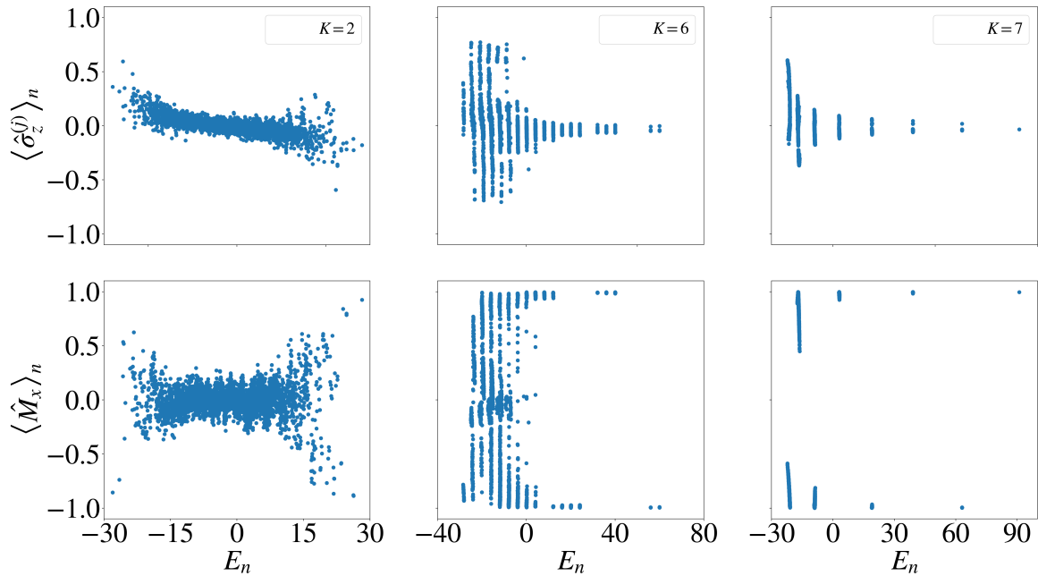
Obrázek 6: Peresovy mříže pro N = 14 a \Delta B = 0,5 . Střední hodnota lokální magnetizace ve směru osy z (nahore) a střední hodnota celkové magnetizace ve směru osy x (dole).
