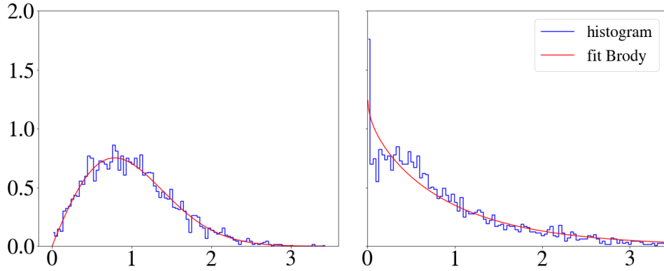
Obrázek 3: Histogram rozdílů sousedních hladin proložený Brodyho rozdělením (1) pro chaotický systém N = 14 , K = 1 , \Delta B = 2,0 s parametrem \beta = 1,0 (vlevo) a nechaotický systém N = 14 , K = 5 , \Delta B = 0,2 s parametrem \beta = 0,0 (vpravo).
