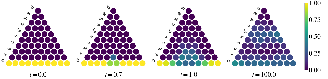
Obrázek 5: Informační mříže pro domain-wall stav řetízku N = 10 s otevřenými okrajovými podmínkami. L = 5 , \Delta B = 0,5 .
