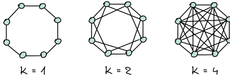
Obrázek 1: Ilustrace stupně propojení K pro N = 8 uzlů s uzavřenými okrajovými podmínkami.
