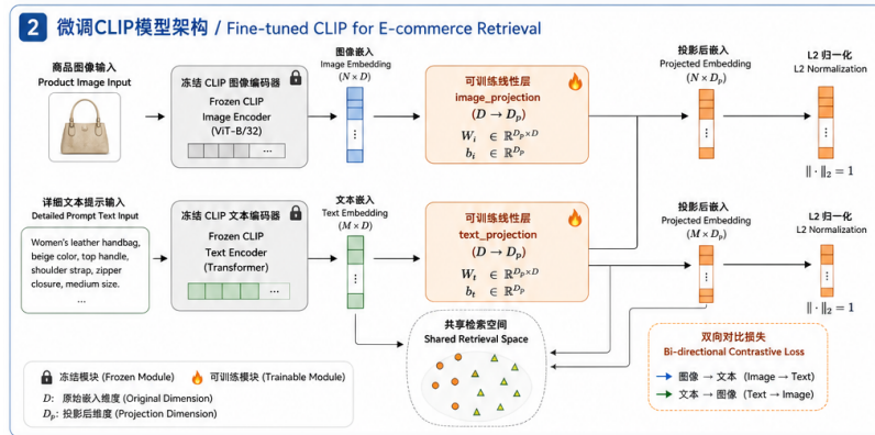
图 2: Linear Probe 微调结构
