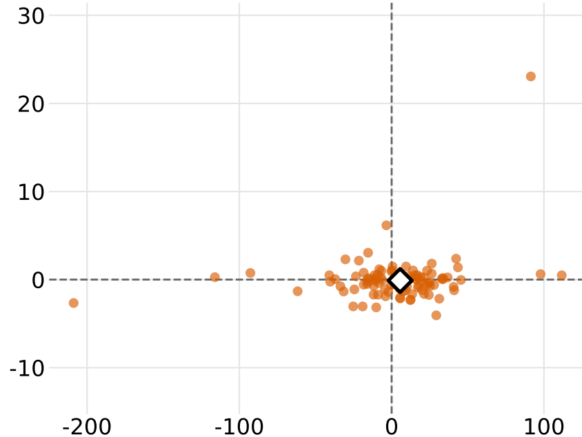
CTDD21 + IF2 warm start (J=100)
