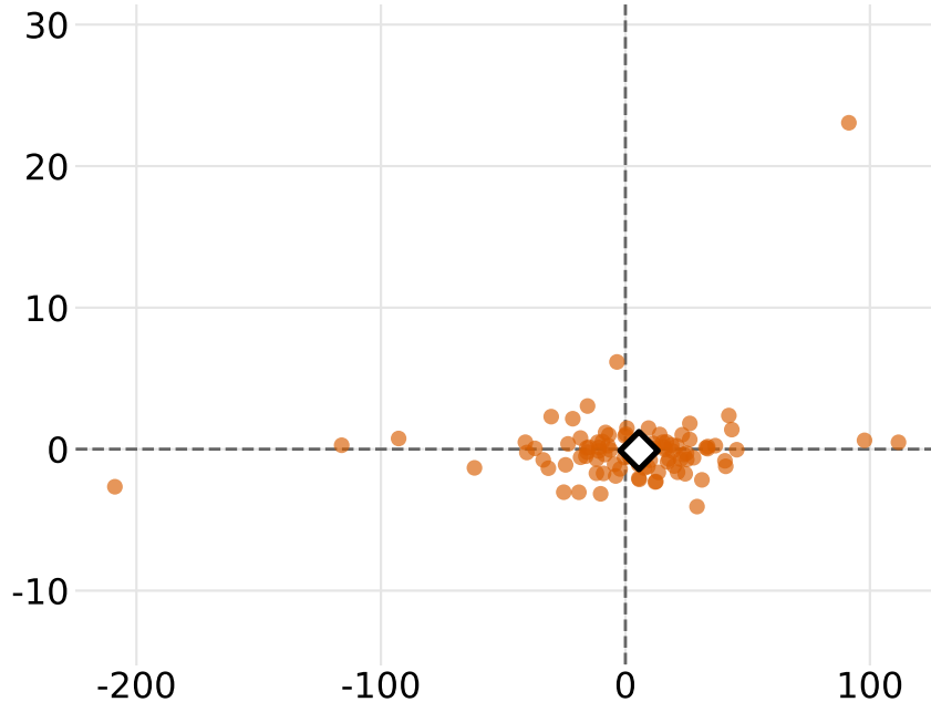
Corenflos + IF2 warm start ( J=100 )
